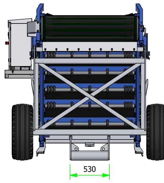
AANZICHT B-B ( 1 : 30 )
