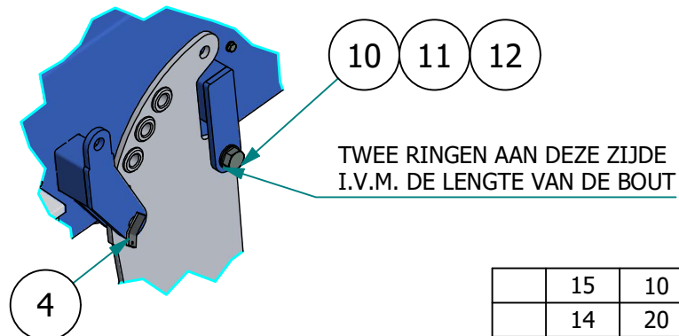
DETAIL D ( 1 : 15 )
