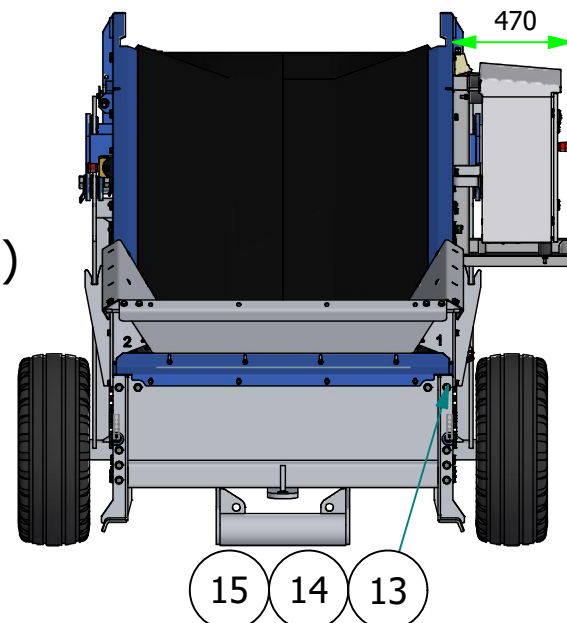
AANZICHT A-A ( 1 : 30 )
