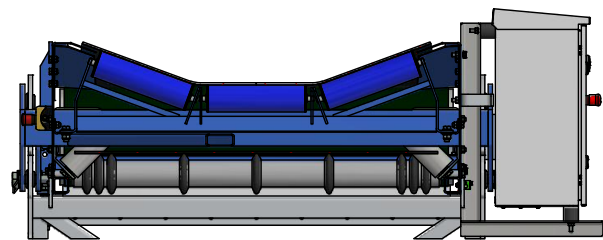
DOORSNEDE E-E ( 1 : 25 )
